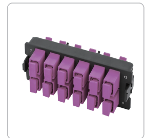
MM(OM4) SC/PC
